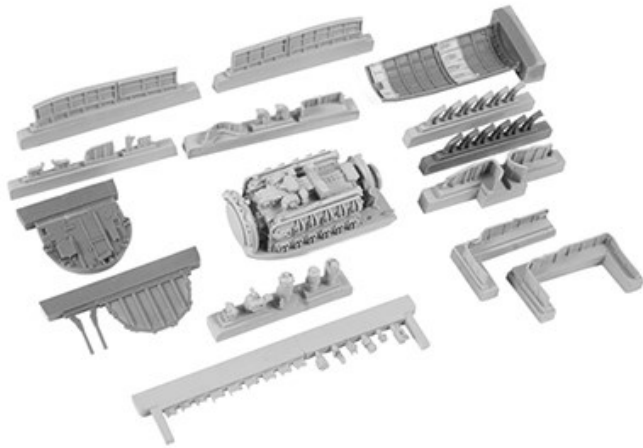
1/48 48CM4393 ホーカーテンペスト・ネピアセイバーエンジン上 部・エデュアルド
