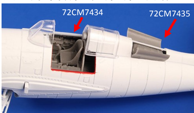
1/72 72CM7434 F4F-4ワイルドキャット・コクピットセット・エアフィクス
