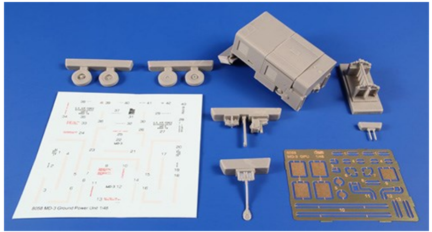
1/48 48CM8058 米空軍・MD-3航空機発電機
