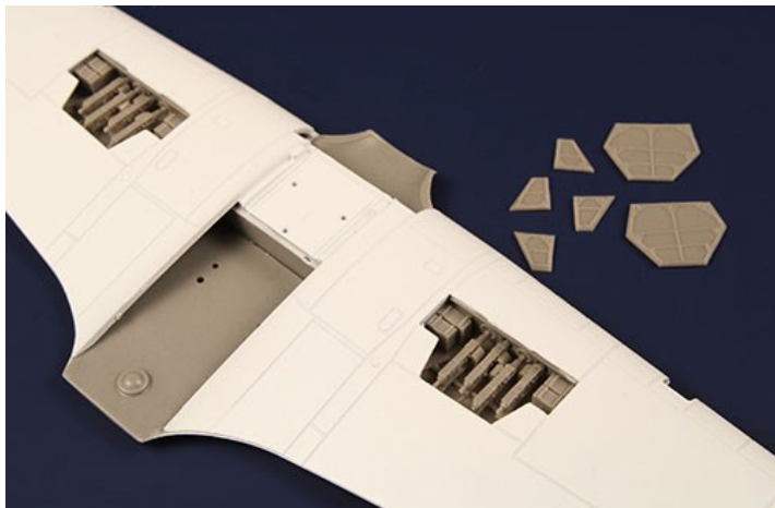
1/72 72CM7451 ホーカーハリケーン用8機銃タイプ主翼機銃点検口
